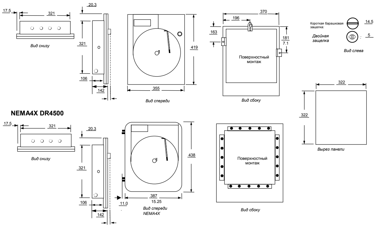
Рис. 3— Размеры самописца DR4500A—только для примера
