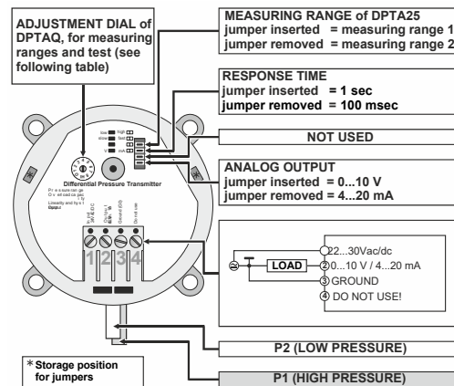
Fig. 3. Wiring details
