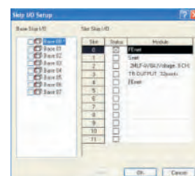
Пропуск входов/выходов
