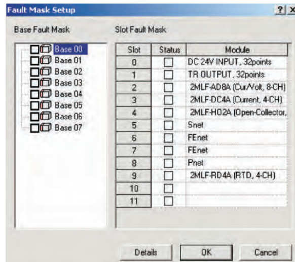
Маскирование ошибок
